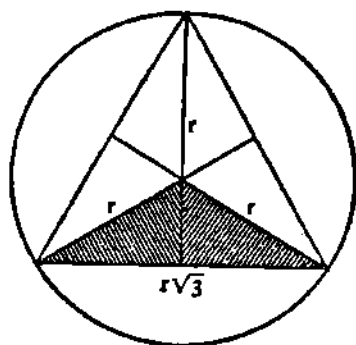
Рис. 2. Платоновский элементарный равносторонний треугольник, составленный из шести субэлементарных неравнобедренных треугольников.
