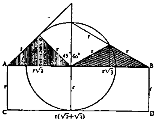
Рис. 3. Прямоугольник ABCD, площадь которого превышает площадь круга менее, чем на 0,15%.
