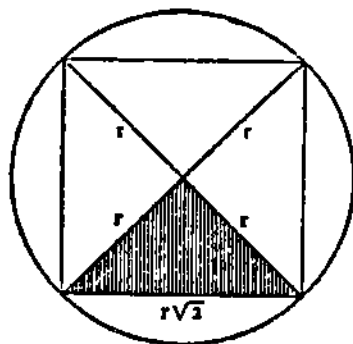
Рис. 1. Платоновский элементарный квадрат, составленный из четырех субэлементарных равнобедренных прямоугольных треугольников.
